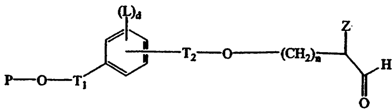
Соединение J
