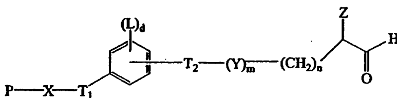
Формула VI
