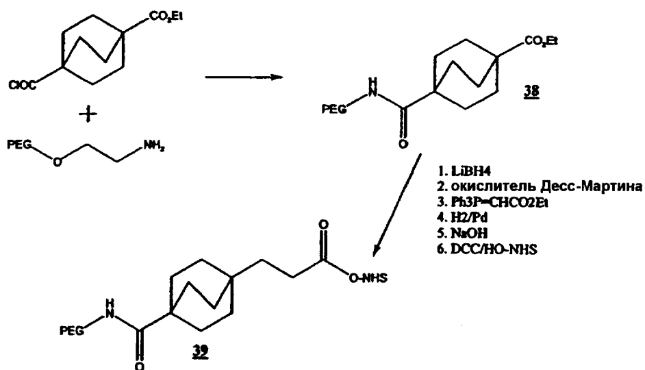
Схема XIV
