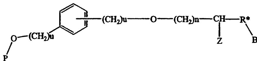
Формула XIX:
