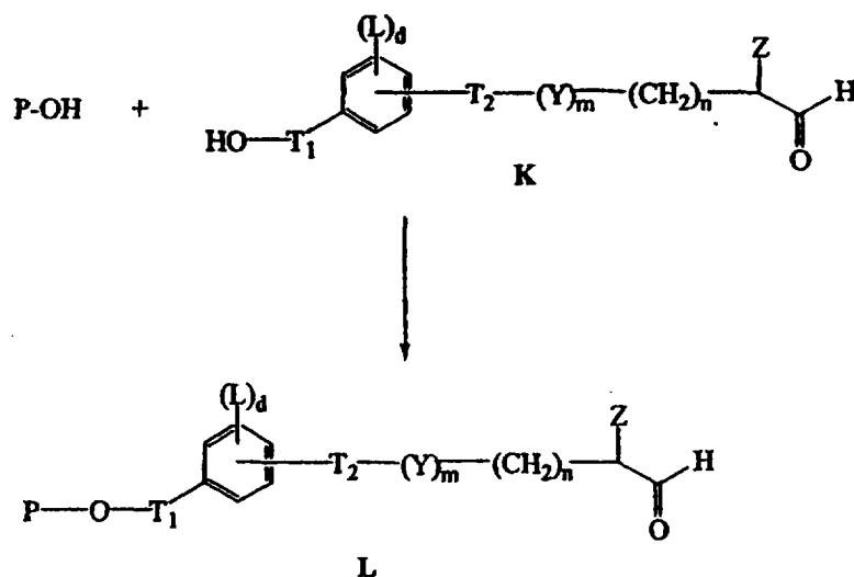
Схема VI:
