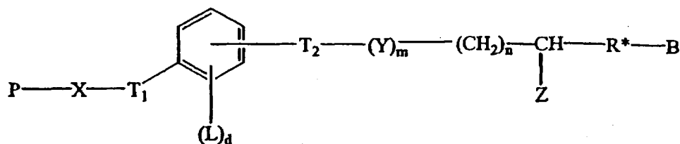
Формула XV
