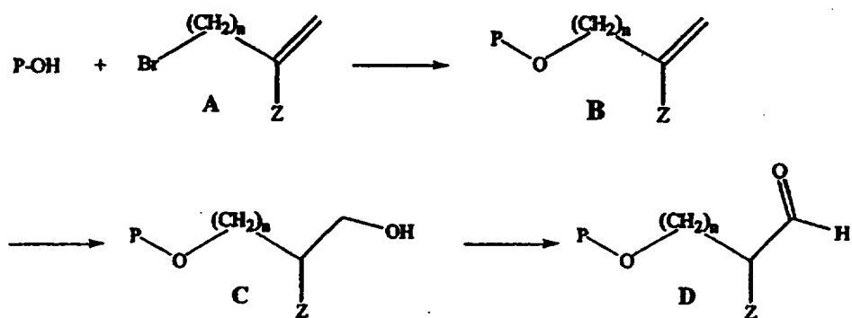
Схема I
