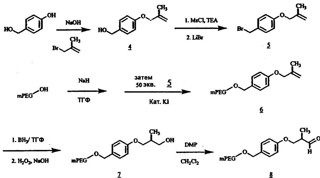
Схема IV:
