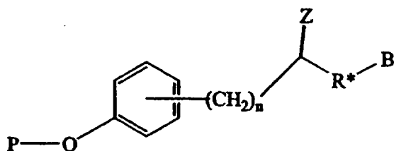
Формула XVII:
