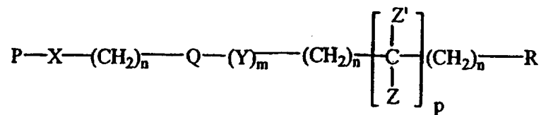
Формула I
