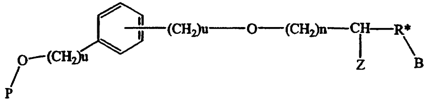
Формула XIX:
