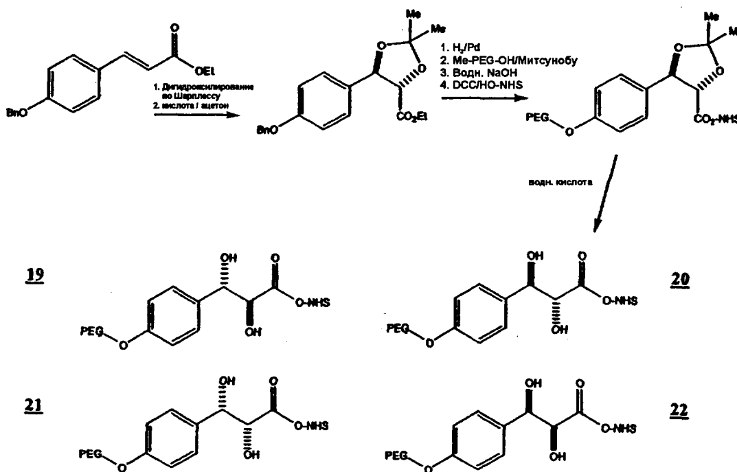
дигидроксидигидроциннамат
