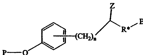
Формула XVIII:
