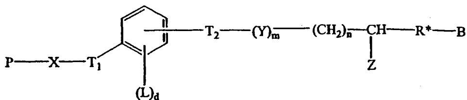
Формула XV:
