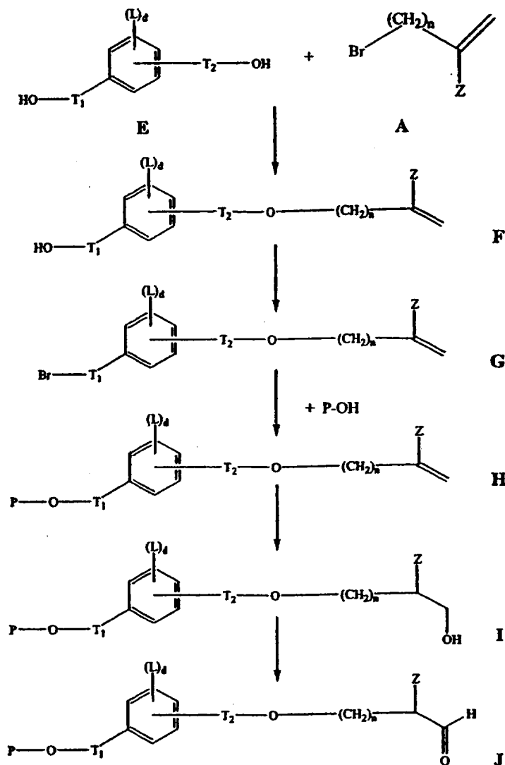
Схема III
