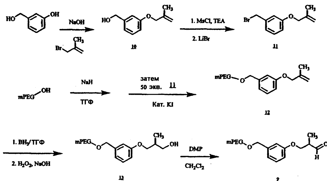
Схема V:
