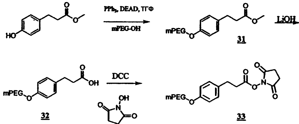
Схема XI
