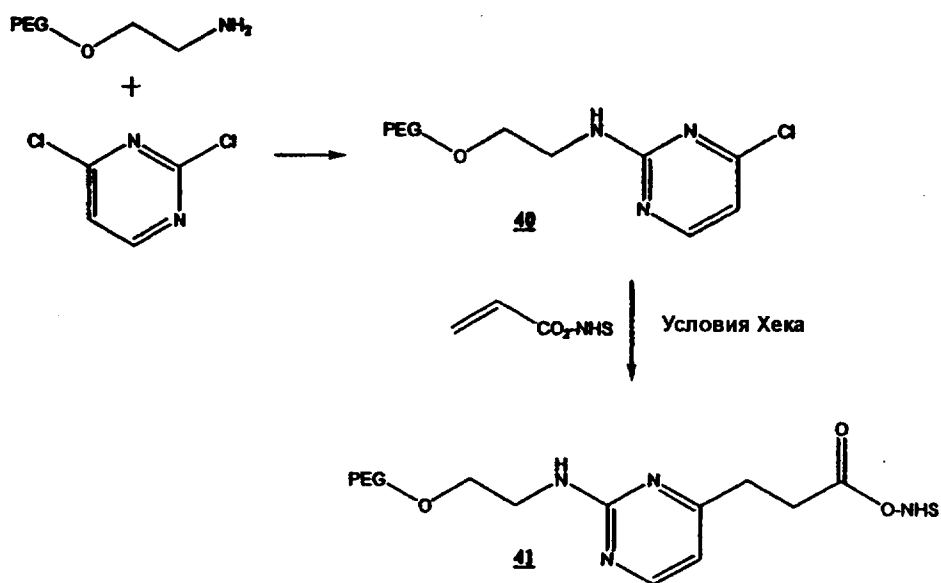
Схема XV
