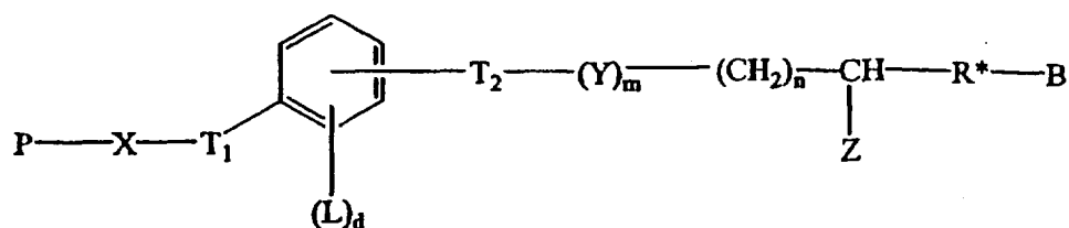
Формула XV:
