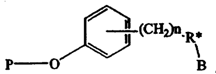
Формула XVIII:
