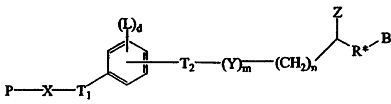
Формула XVI:
