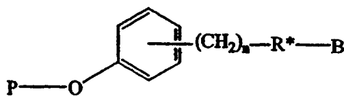
Формула XVIII:
