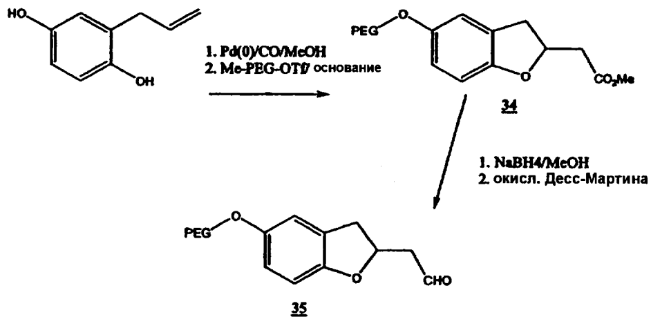
Схема XIII
