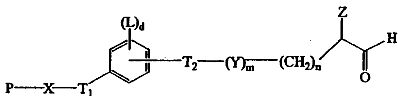
Формула VI
