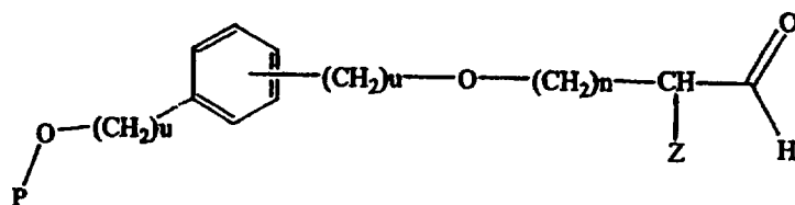
Формула IX:
