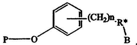
Формула XVIII:
