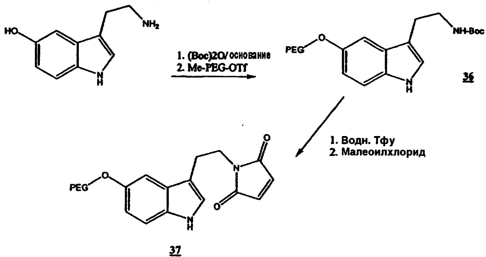
Схема XIII
