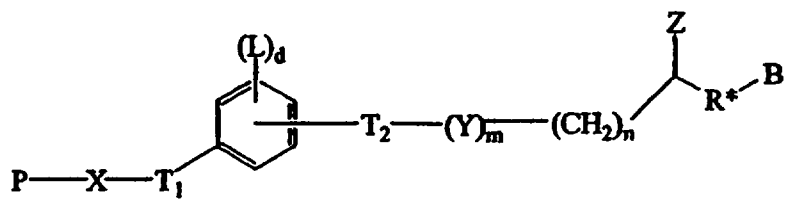
Формула XVI
