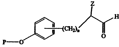
Формула VIII:
