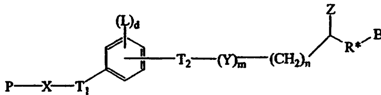
Формула XVI
