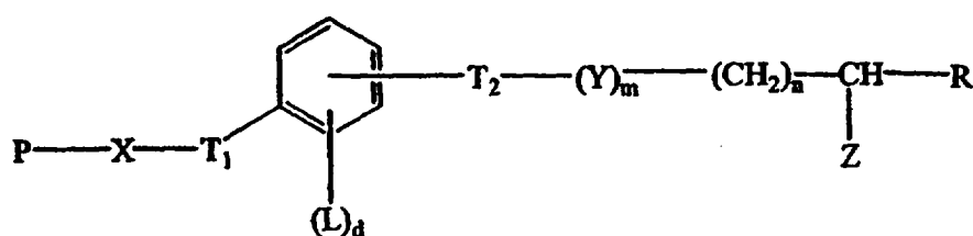
Формула V
