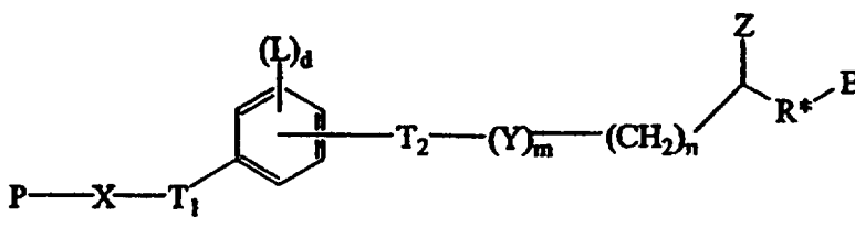
Формула XVI
