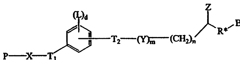
Формула XVI
