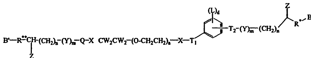
Формула XX:
