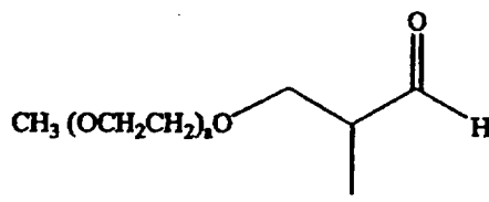
Формула XIII:
