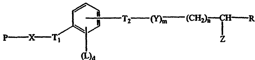
Формула V
