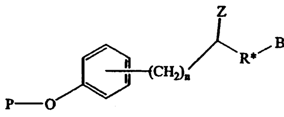
Формула XVII:
