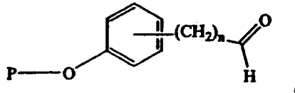
Формула VIII:
