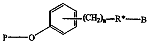
Формула XVIII:
