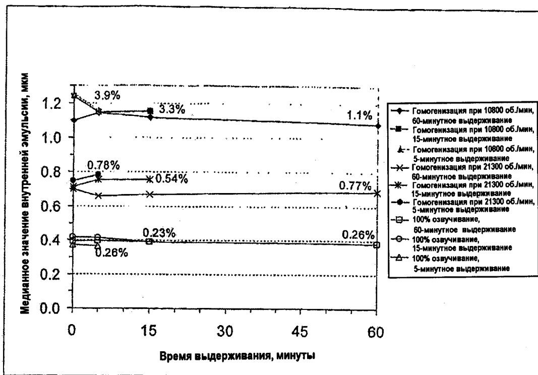
Фиг. 9
