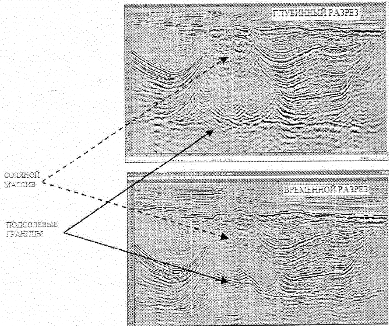
Рисунок 1. Глубинный (сверху) и временной (снизу) разрезы, полученные с использованием попластового скоростного анализа по исходным сейсмограммам без использования данных гравirazведки.
