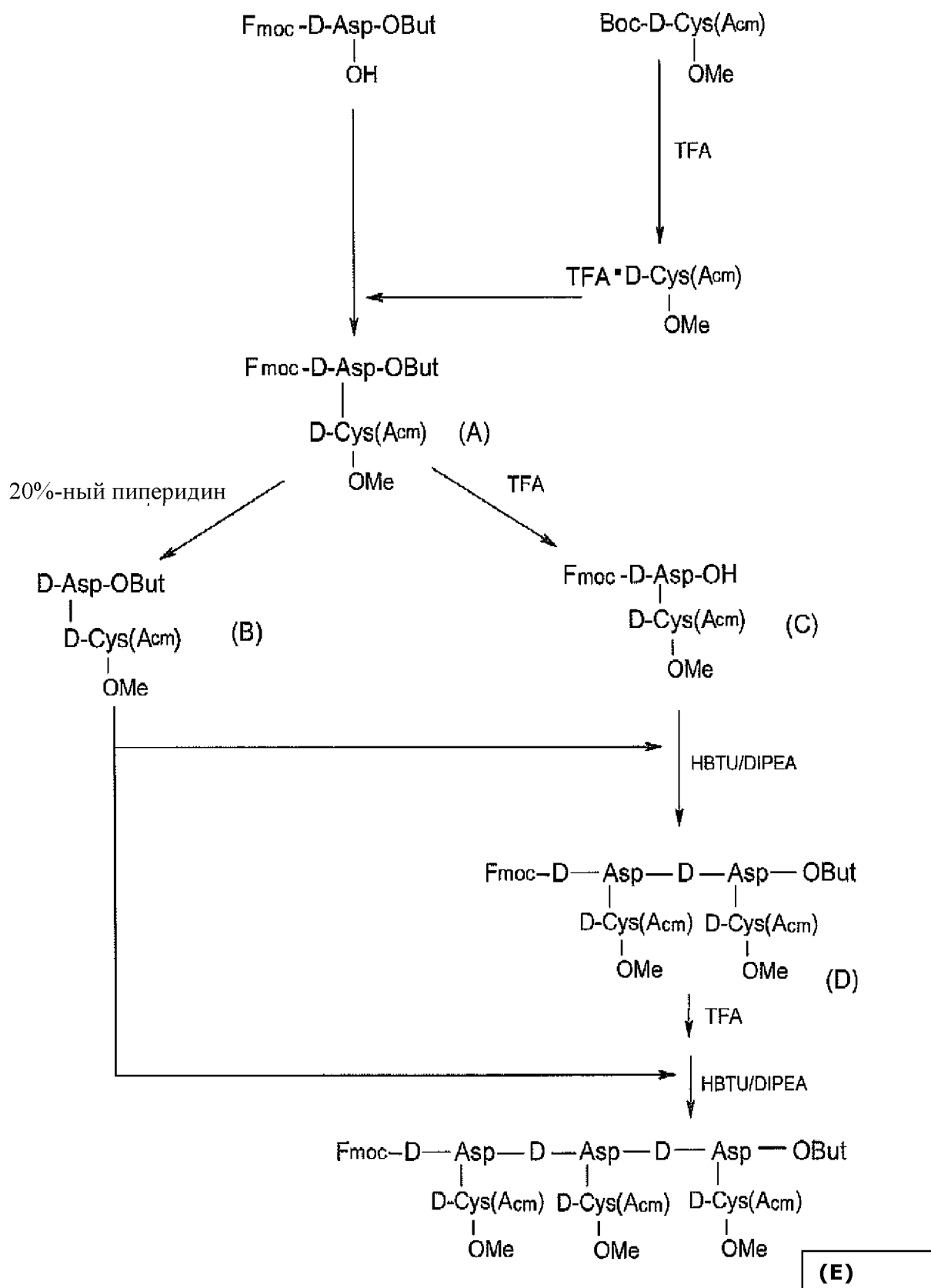
Схема 15: Получение кислотной/анионной группы D-Asp(D-Cyst)-D-Asp(D-Cyst)-D-Asp(D-Cyst)-OH
