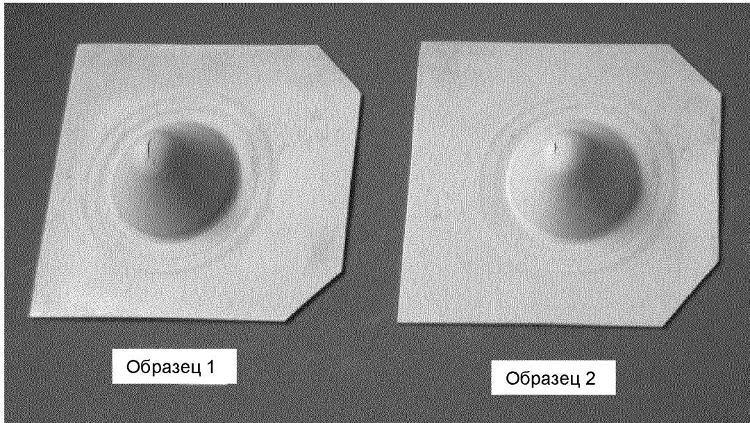
Образец № 1 (слева) и № 2 (справа) сплава №1 после испытания на способность к формоизменению
