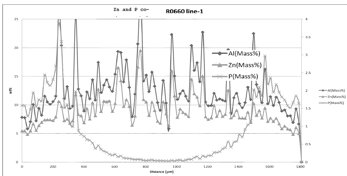
Фигура 1: Графики концентраций цинка, фосфора и алюминия по всему экструдату, измеренные с использованием сканирующего электронного микроскопа с дисперсионным рентгеновским спектральным анализом. Образец подготавливают посредством одновременной пропитки водным раствором \text{Zn}(\text{NO}_3)_2 и \text{H}_3\text{PO}_4 .
