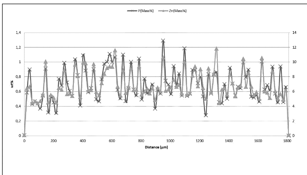
Фигура 2: Графики концентраций цинка и фосфора по всему экструдату, измеренные с использованием сканирующего электронного микроскопа с дисперсионным рентгеновским спектральным анализом. Носитель готовят посредством добавления \text{H}_3\text{PO}_4 перед выполнением экструзии (вместе с ZSM-5, оксидом алюминия и др.). Носитель пропитывают водным раствором \text{Zn}(\text{NO}_3)_2 .
