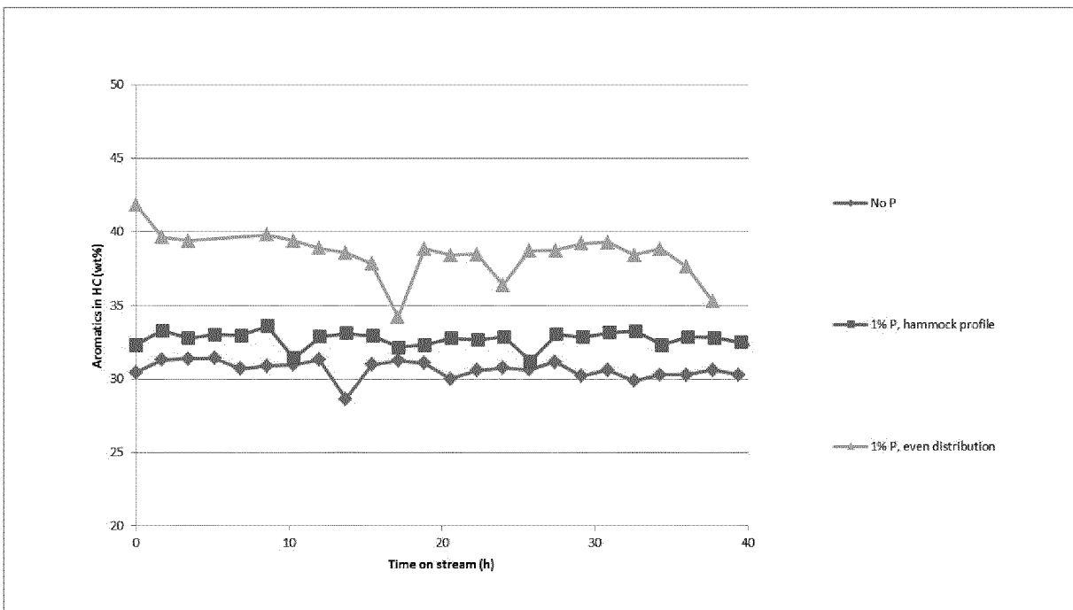
Фигура 3: Мас.% ароматических соединений для обработанных паром катализаторов (500 °С, 48ч). Все катализаторы пропитывают 10 мас.% цинком.
