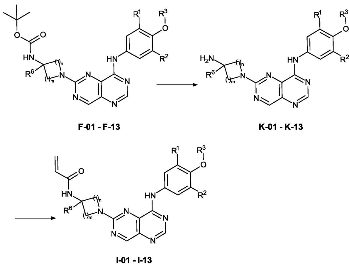
Схема 4а. Синтез соединений I-01 – I-13
