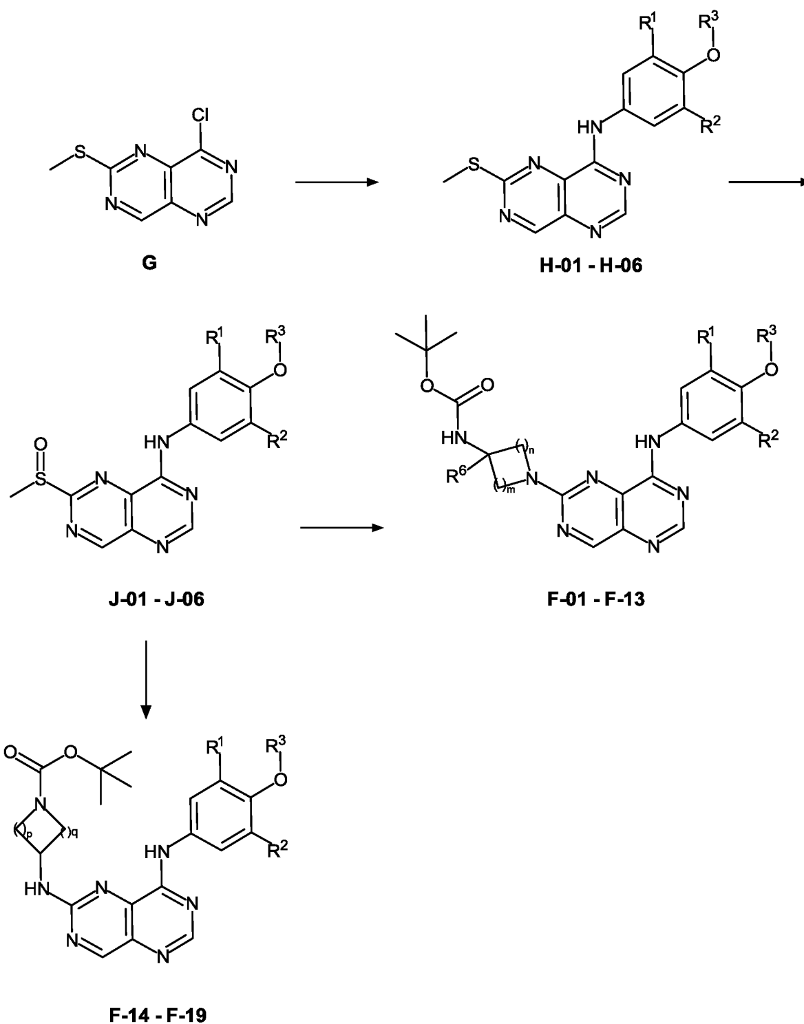
Схема 3. Общий способ 2 для синтеза соединений F-01 – F-19
