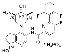
Соль фосфорной кислоты Соединения 1
