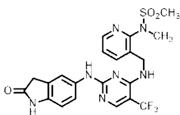
Формула (I-e)
