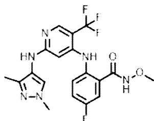
Формула (I-f)
