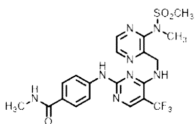
Формула (I-d)
