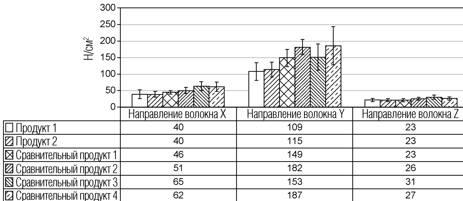
Сжатие влажного синтетического волокнистого продукта
