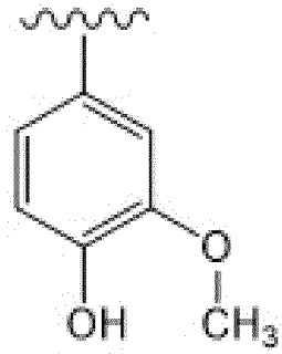
гвайацил (S)
