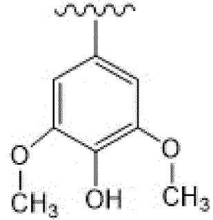
сирингил (S)
