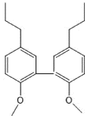
5\text{-5'}
