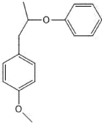
\beta\text{-O-4'}
