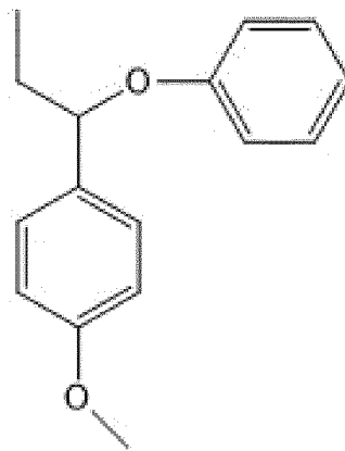
\alpha\text{-O-4'}
