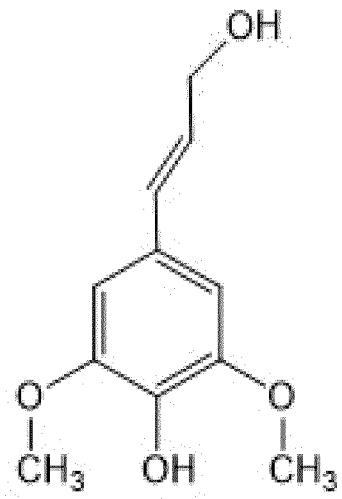
синапил
