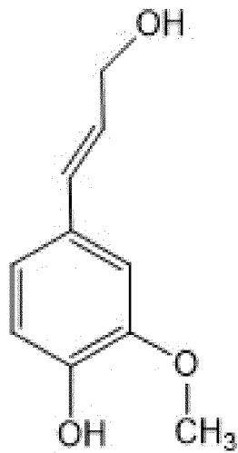
коницерил
