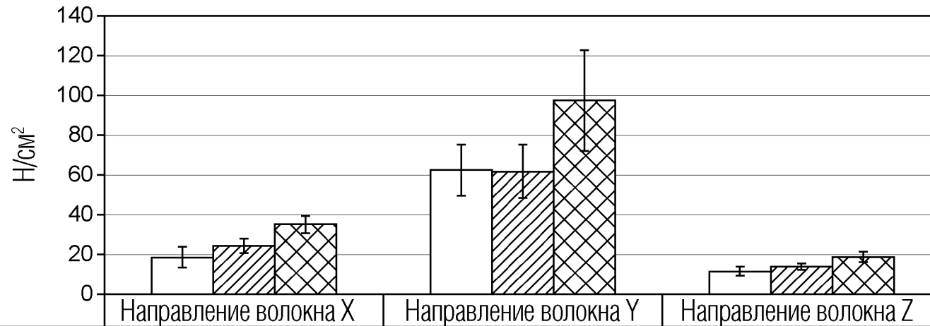
Сжатие влажного волокнистого продукта
