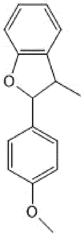
\beta\text{-5'}
