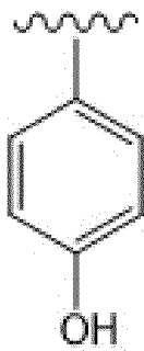
пара-гидроксифенил (H)
