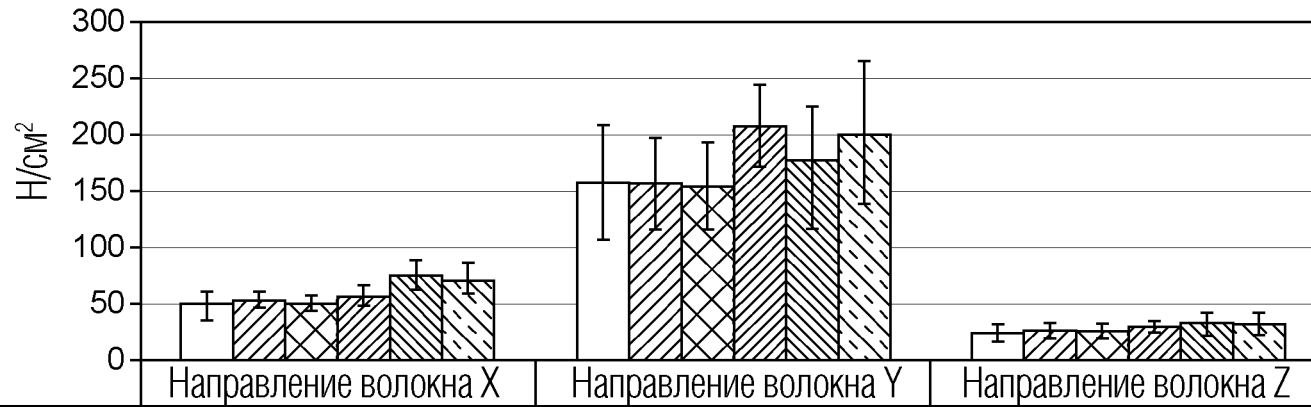
Сжатие сухого синтетического волокнистого продукта
