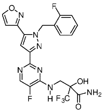
Формула IV
