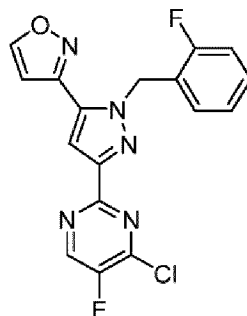
Формула VI
