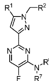
Формула IV
