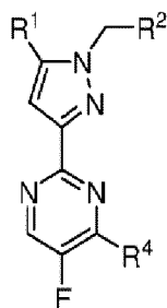
Формула I
