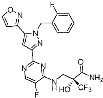
Формула ID
