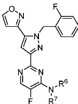
Формула VII
