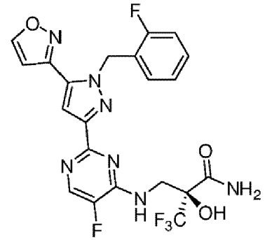
Формула IC
