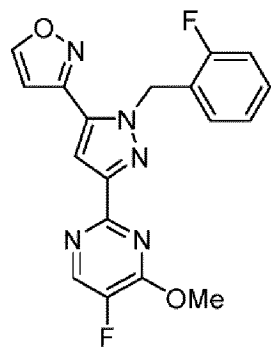
Формула V
