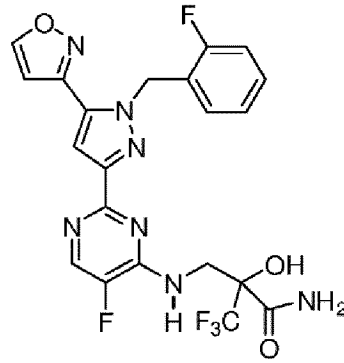
Формула IB
