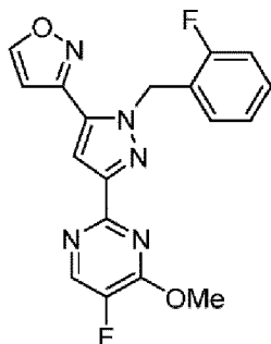
Формула V
