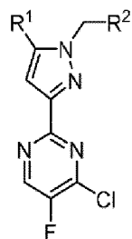
Формула III
