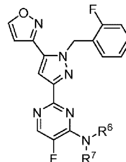
Формула VII
