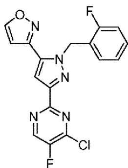
Формула VI
