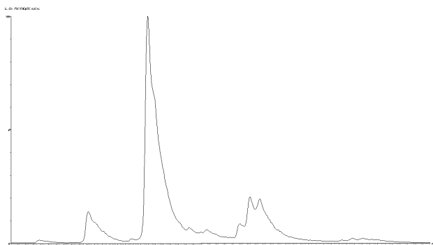
В) Свернутый спектр MS для образца для трансфекции ZO (T366K/L351'D). Второй/главный пик соответствует биспецифической молекуле.
