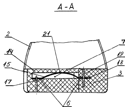
Фиг. 2б Разрез
