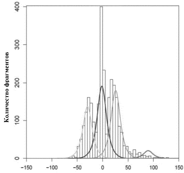
z-показатель Фиг. 10В
