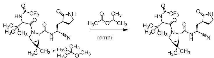
13, сольват метил-трет-бутилового простого эфира
