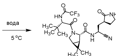
13, сольват метил-трет-бутилового простого эфира
