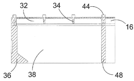
Разрез В-В Фиг. 10С
