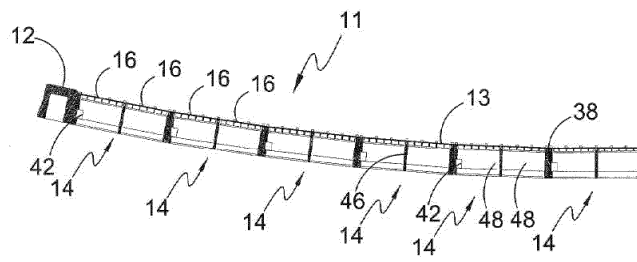
Разрез А-А Фиг. 7А
