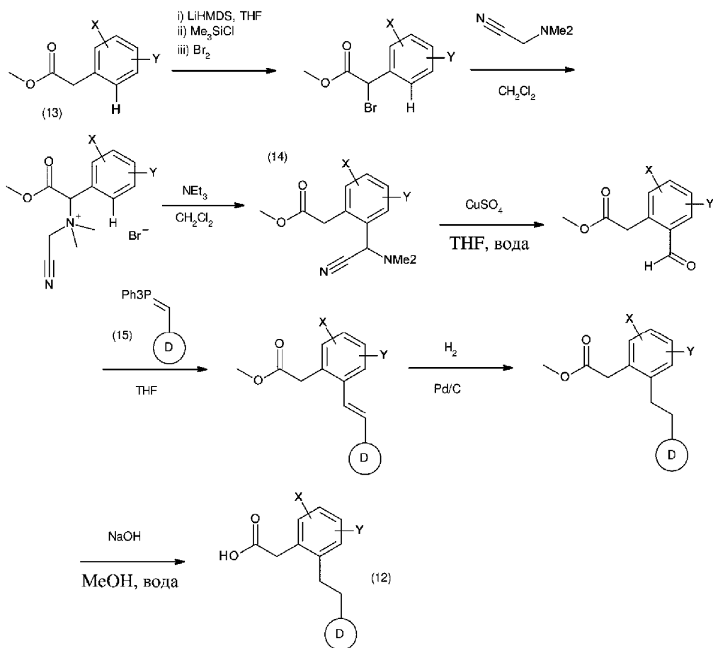
Схема реакции 9.
