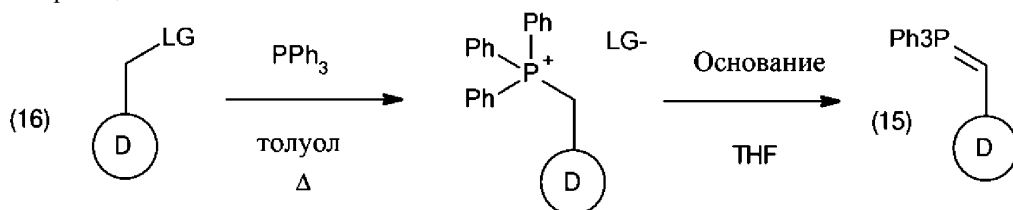
Схема реакции 9.
