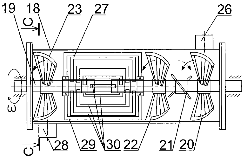
Вид С
