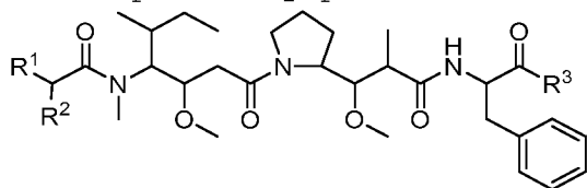
Формула (A),
