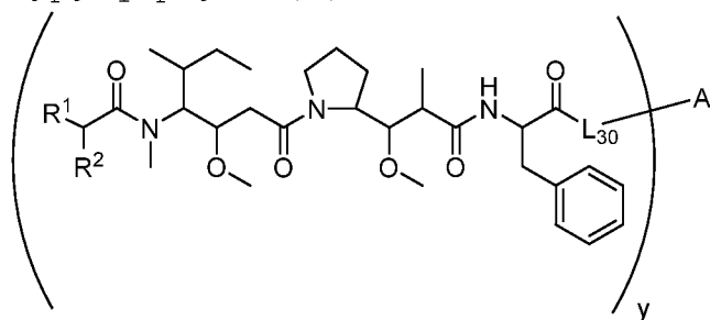
Формула (D),
