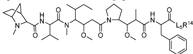
Формула (А-2),
