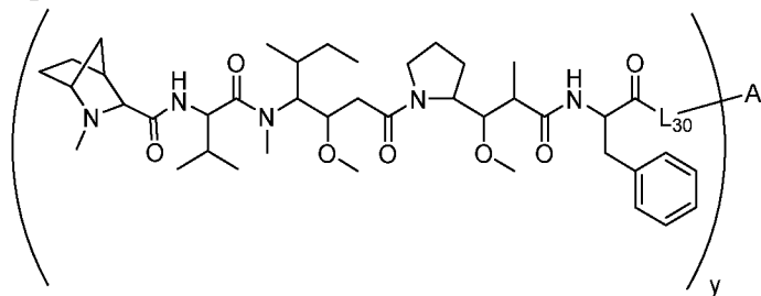
Формула (D-1),
