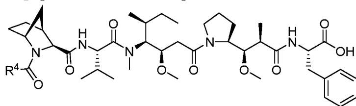
Формула (А-1а),
