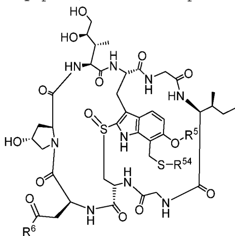
Формула (B-1a),
