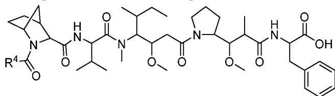
Формула (А-1),
