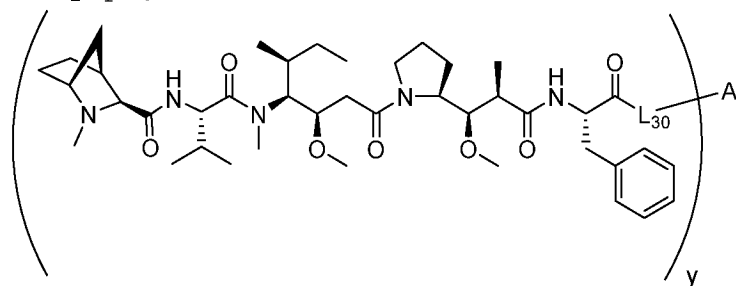
Формула (D-1a),
