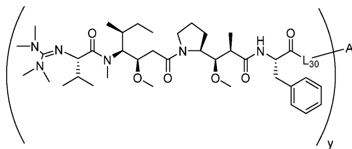
Формула (D-2a),
