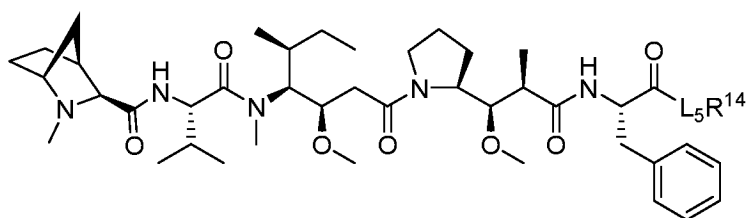
Формула (А-2а),
