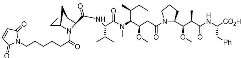
(C2)
