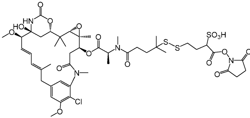
(сульфо-SPDB-DM4)
