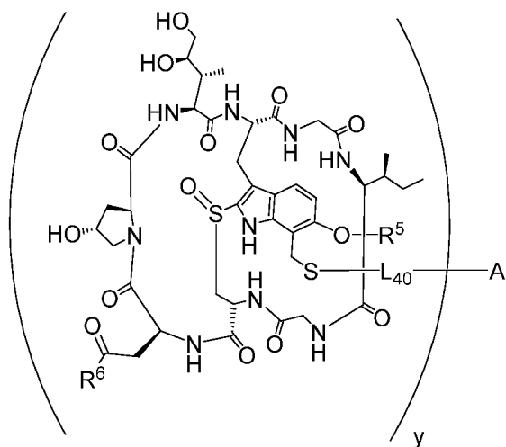
Формула (E-1a),
