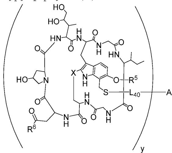
Формула (E),
