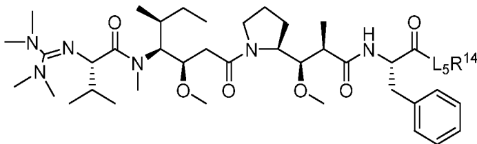
Формула (А-3а),
