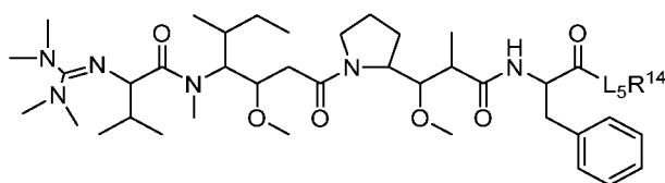
Формула (А-3),
