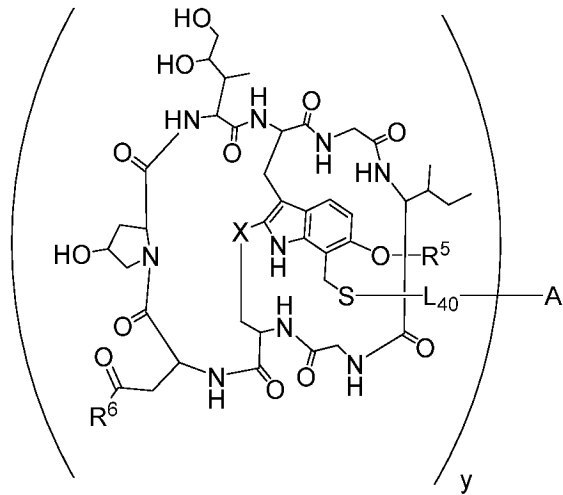
Формула (E),
