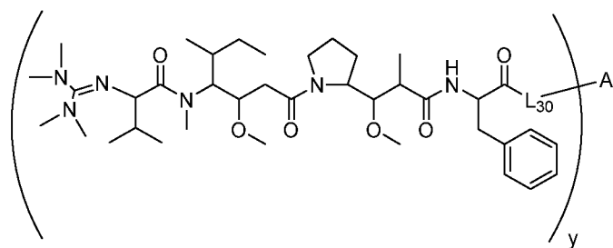
Формула (D-2),
