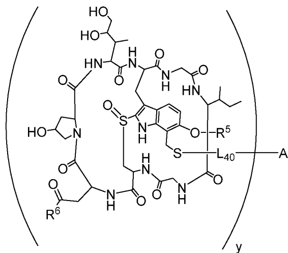
Формула (Е-1),
