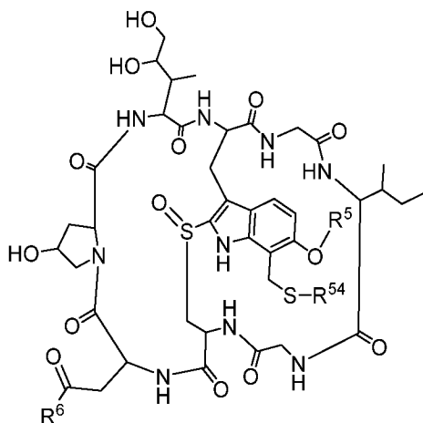
Формула (B-1),
