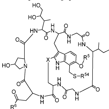
Формула (B),
