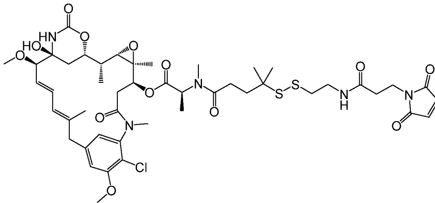
(MPET-DM4).
