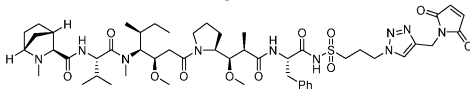
(С3)
