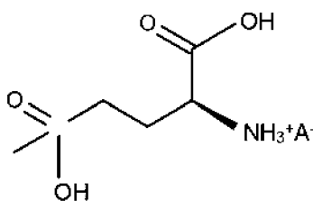
Формула (II)
