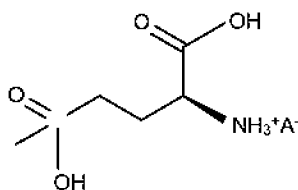
Формула (II)
