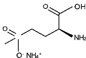
Формула (I),
