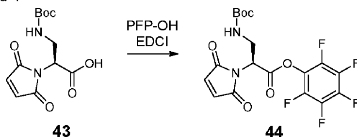
Схема 4
