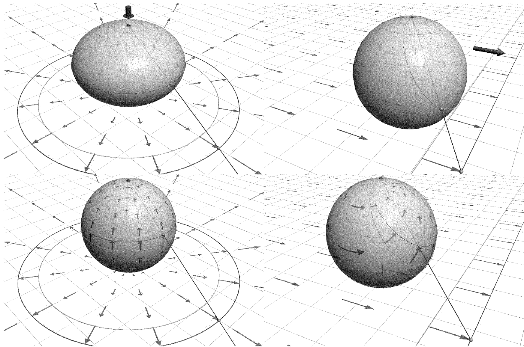
Фигура 2. Построение дифференциальных движений сферы с помощью стереографической проекции.
