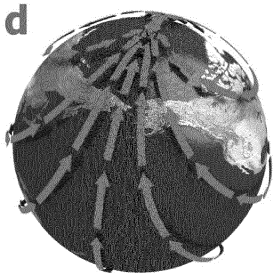
Фигура 3. Элементы расширенной группы движений Земли с учётом дифференциальных вращений.
