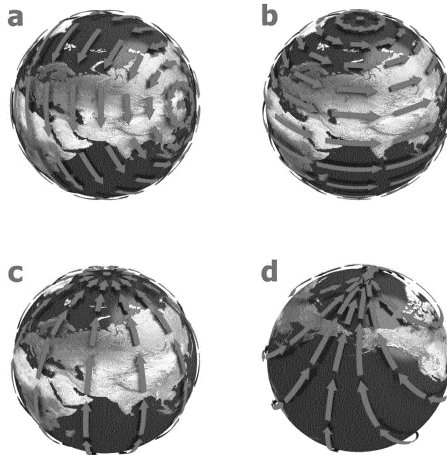
Элементы расширенной группы движений Земли с учётом дифференциальных вращений.
