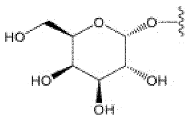
альфа-d-галактоза
