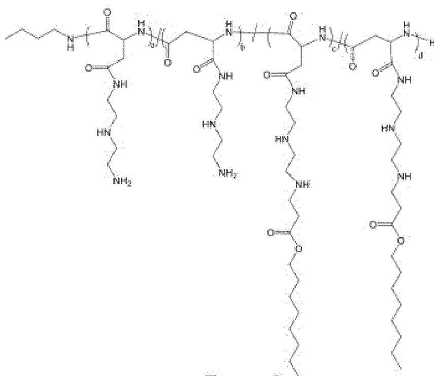
Полимер 8
