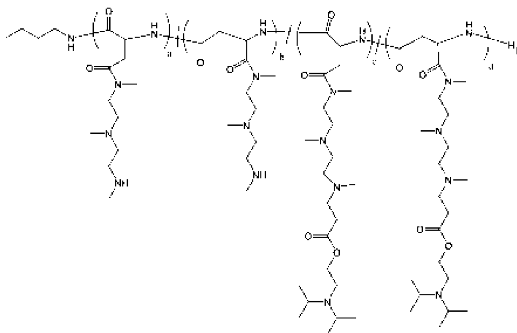
Полимер 15
