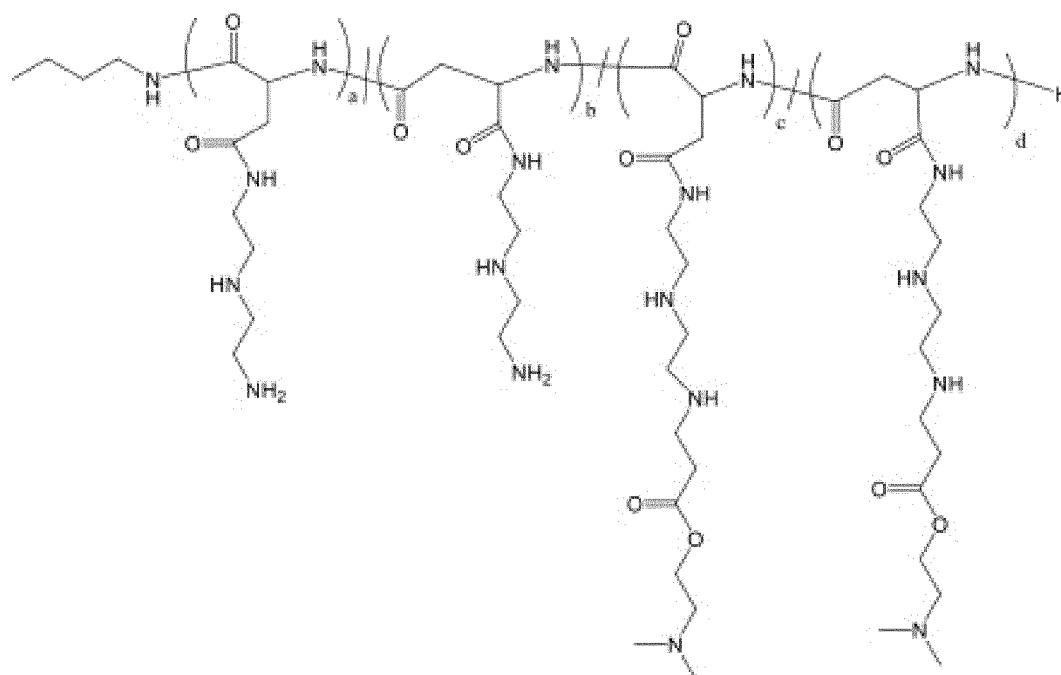
Полимер 1
