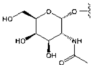
N-ацетилгалактозамин
