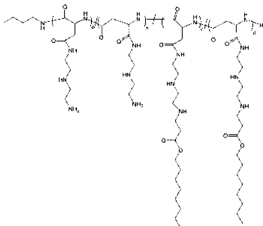
Полимер 8
