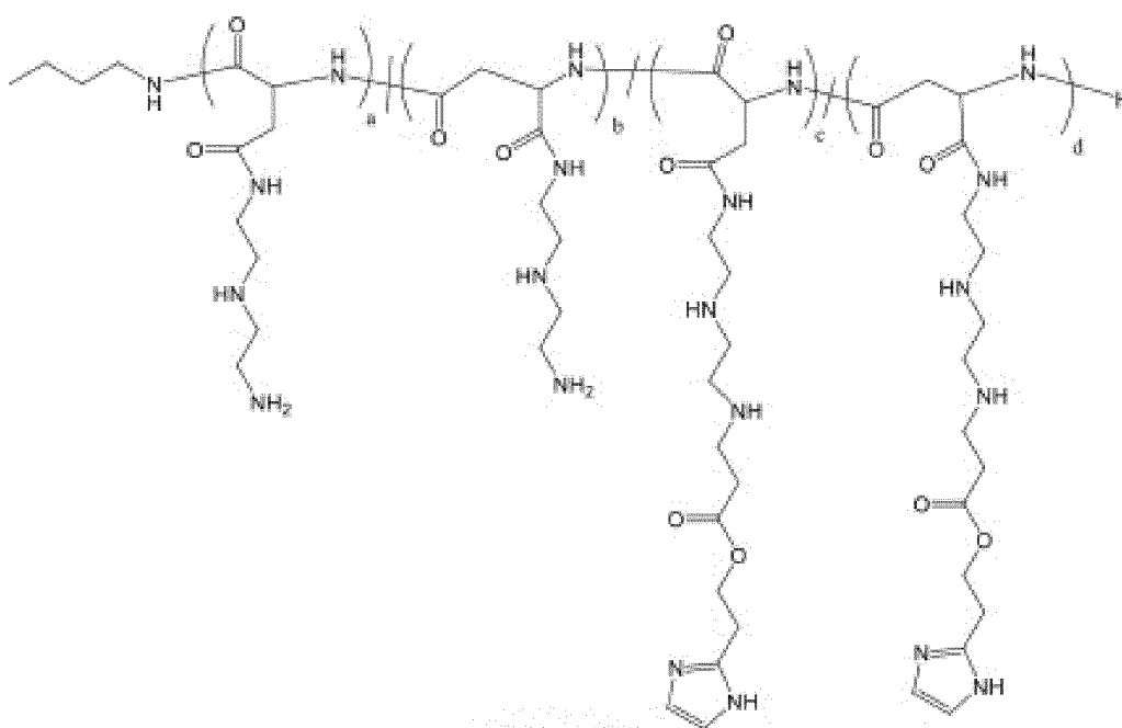
Полимер 6
