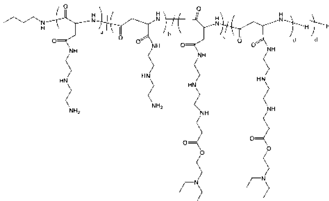
Полимер 2
