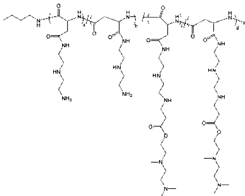
Полимер 5
