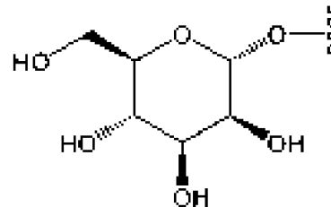
альфа-d-манноза
