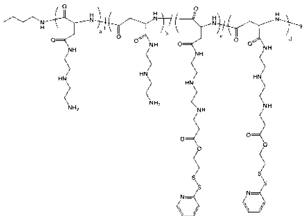
Полимер 4
