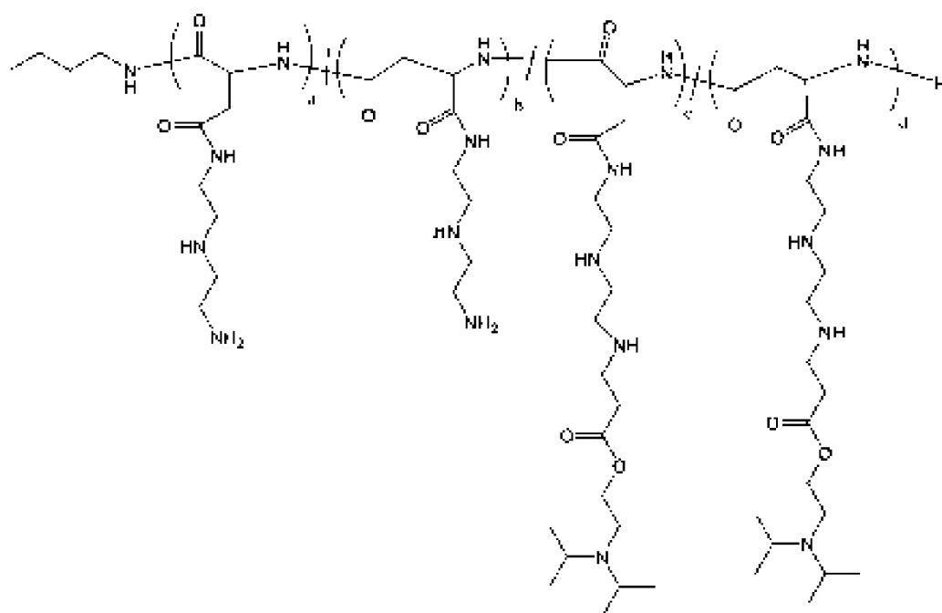
Полимер 3
