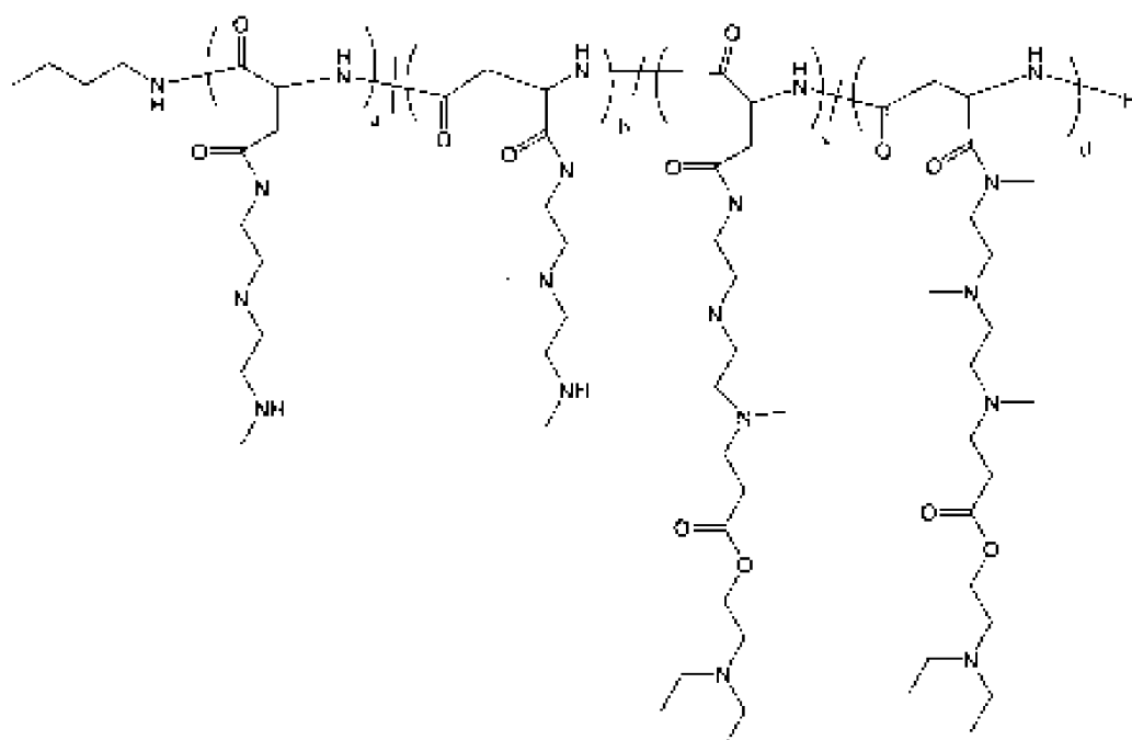
Полимер 14
