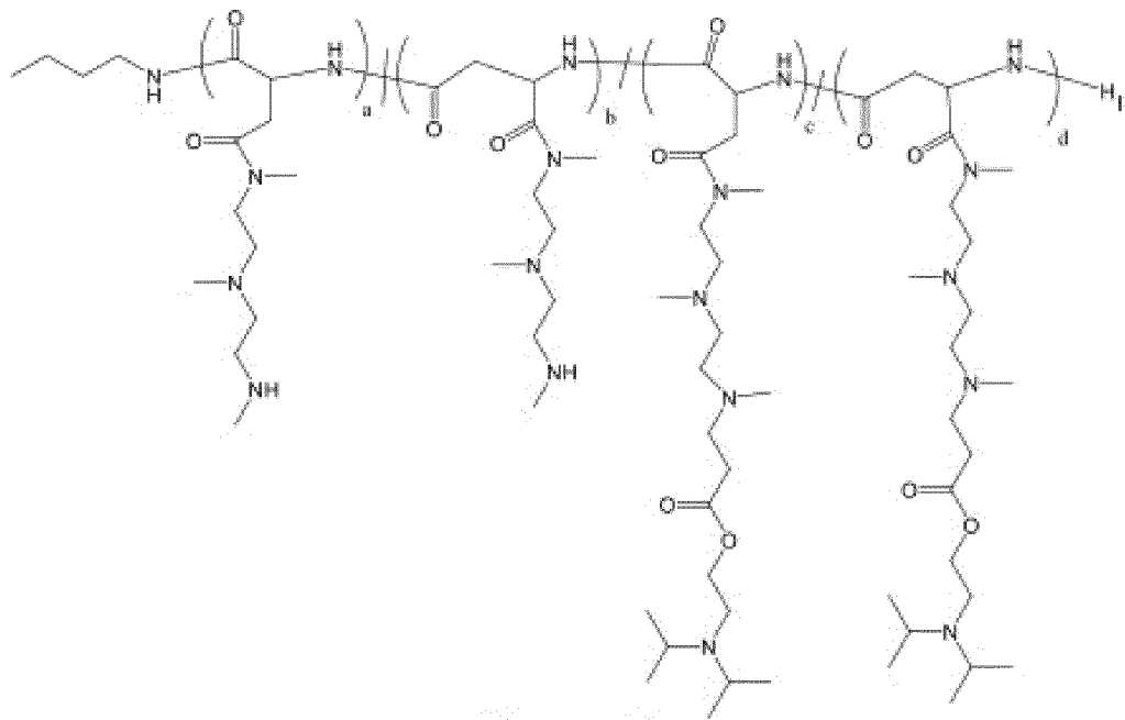
Полимер 15
