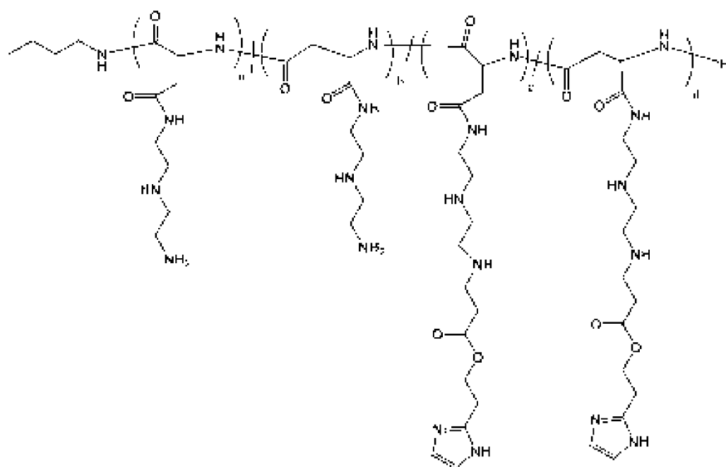
Полимер 6
