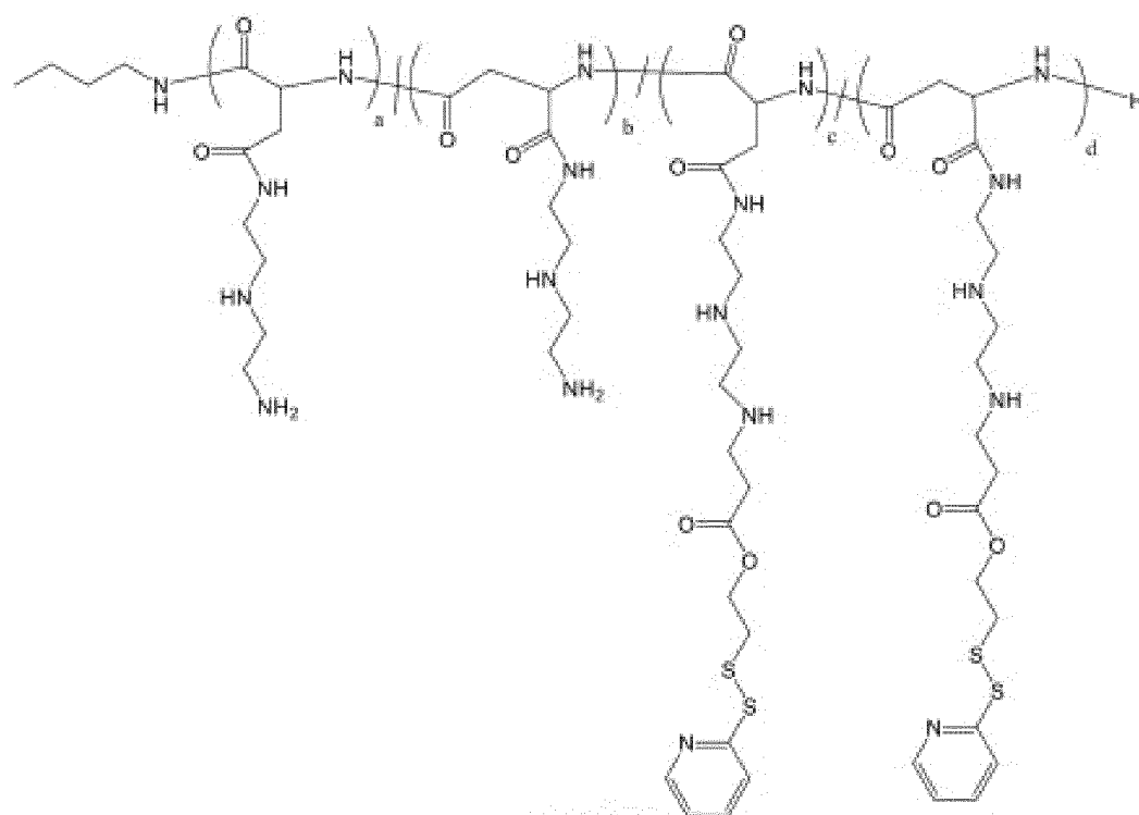
Полимер 4
