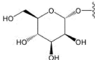
альфа-d-манноза
