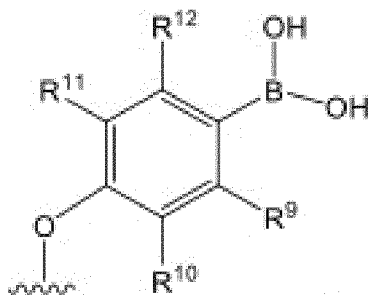
фенилборная кислота
