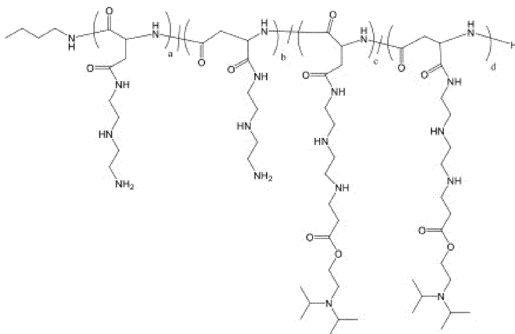
Полимер 3
