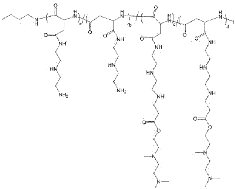
Полимер 5
