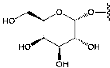
альфа-d-галактоза
