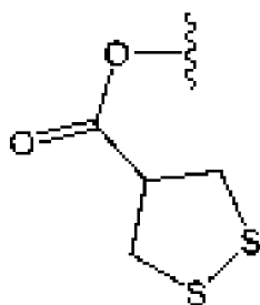
спаржевая кислота
