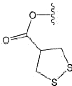
спаржевая кислота
