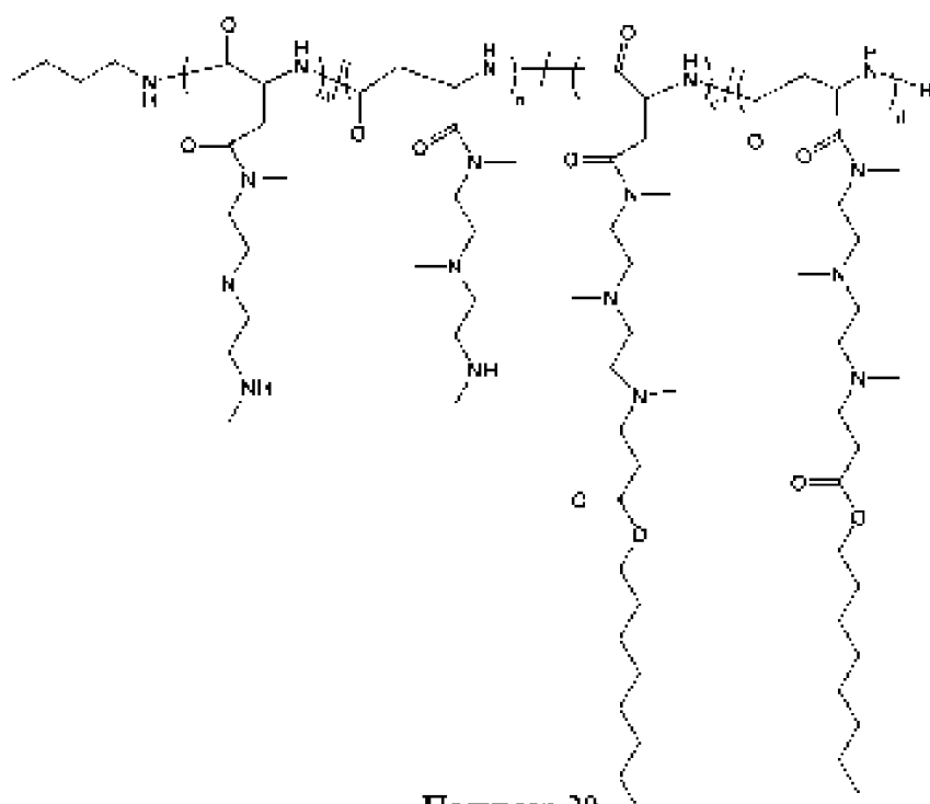
Полимер 20
