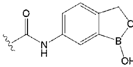
фенилборная кислота
