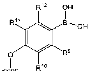
фенилборная кислота
