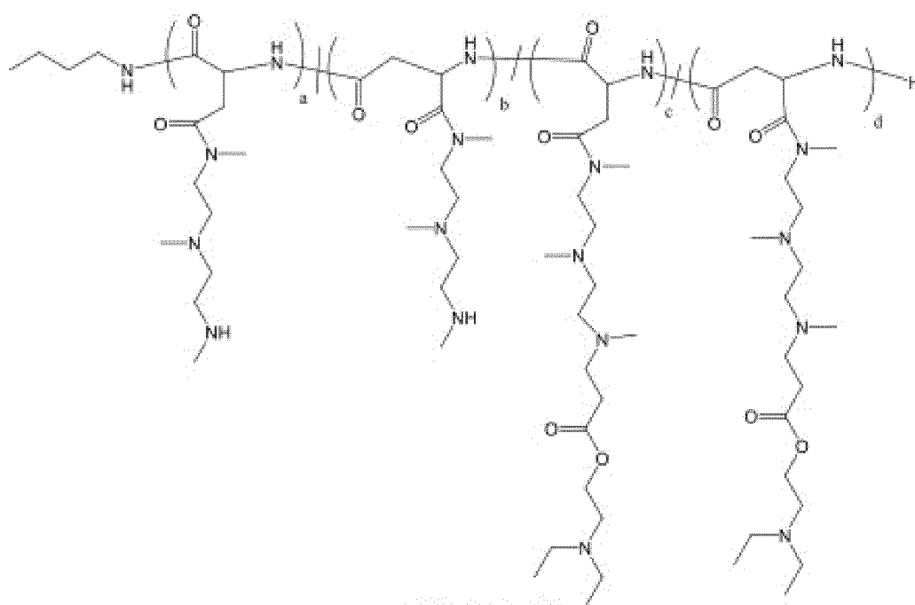
Полимер 14
