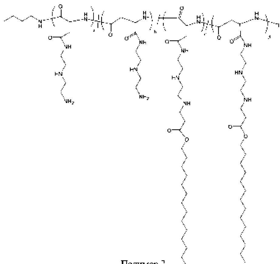
Полимер 7
