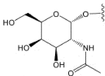
N-ацетилгалактозамин
